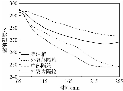
图 9 爬升与巡航阶段各隔舱的燃油温度
