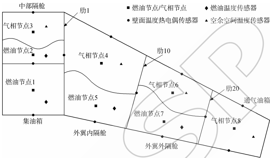
图 1 油箱结构示意图 Fig. 1 Structure diagram of fuel tank
