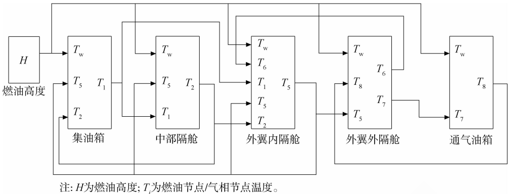
图 4 基于 Simulink 的油箱热力学模型框架 Fig. 4 Fuel tank thermodynamic model framework based on Simulink
