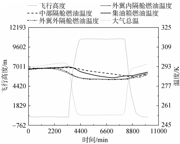
图 11 各隔舱燃油温度变化规律(标准天短航程)
