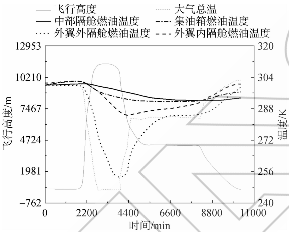
图 12 各隔舱燃油温度变化规律(热天短航程)
