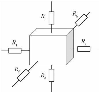
图 2 节点热阻示意图 Fig. 2 Schematic diagram of node thermal resistance
