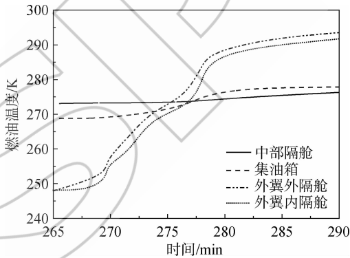
图 10 下降阶段各隔舱燃油温度规律
